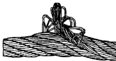
Рисунок 11. Выдавливание сердечника
