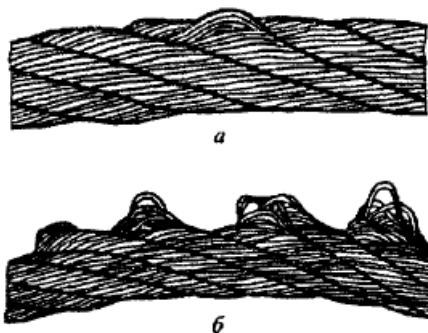
Рисунок 12. Выдавливание проволок прядей: а - в одной пряди; б - в нескольких прядях
