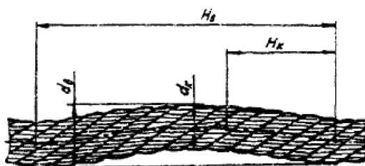
Рисунок 9. Волнистость каната
